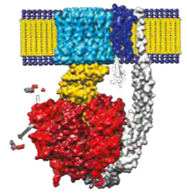
2 Modell der ATP-Synthase
