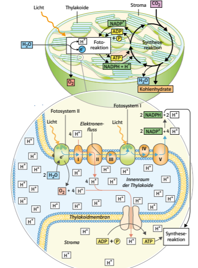
1 Chemiosmotisches Modell der ATP-Bildung
